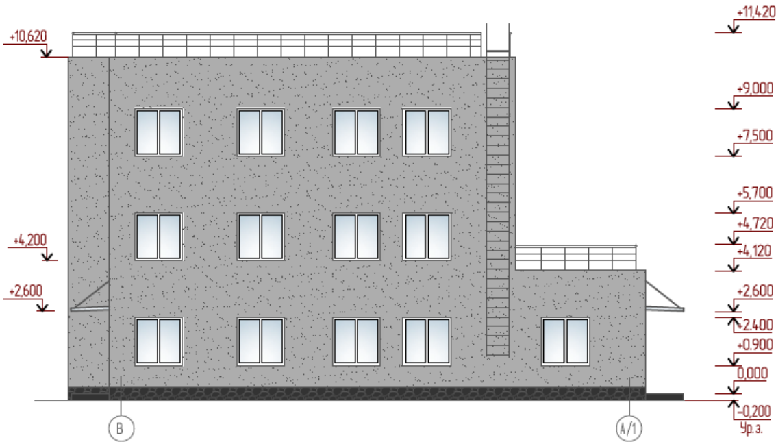
Фасад В - А/1
