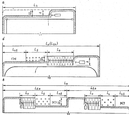
Рис. 3.12. Схемы разделения блоков панели на рабочие блоки: L_n ( L_n ), L_б и L_{н.б} — длина взорванного (экскавируемого), бурового и подготовленного к бурению блоков; 1 — забойный путь
